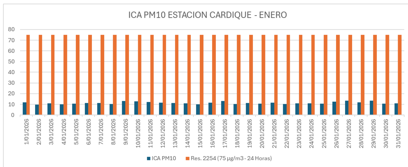
Gráfico 2. Concentración promedio de PM10 EST. CARDIQUE
