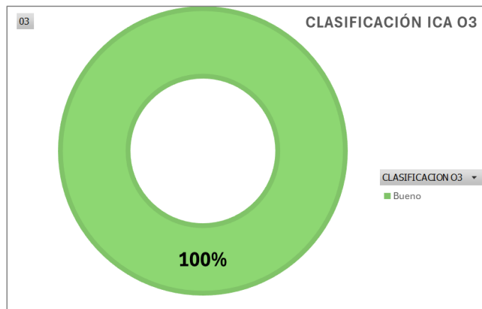
Gráfico 10. Índice de Calidad del Aire O 3 BOCANA
