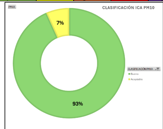
Gráfico 7. Índice de Calidad del Aire PM 10 MAMONAL
