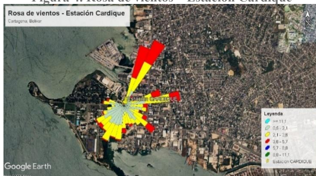
Figura 4. Rosa de vientos – Estación Cardique
