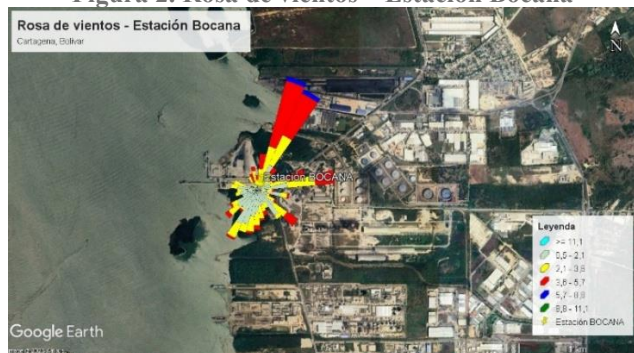
Figura 2. Rosa de vientos – Estación Bocana
