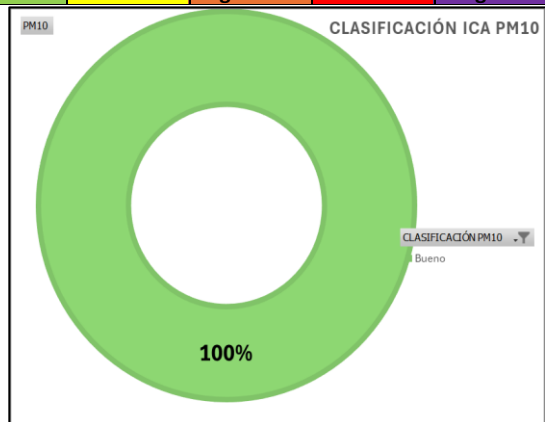
Gráfico 6. Índice de Calidad del Aire PM 10 CARDIQUE
