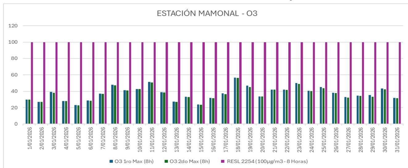
Gráfico 5. Concentración promedio de O 3 EST. MAMONAL
