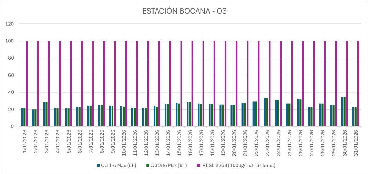
Gráfico 3. Concentración promedio de O 3 EST. BOCANA
