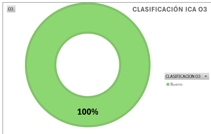
Gráfico 8. Índice de Calidad del Aire O 3 CARDIQUE
