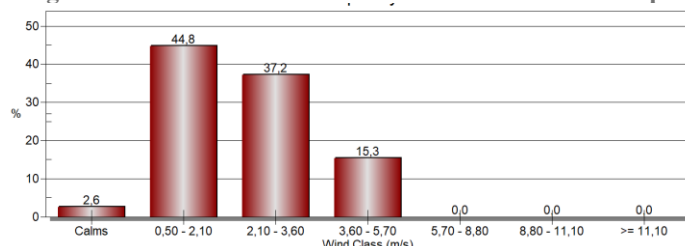
Figura 5. Distribución de frecuencia de vientos - Cardique
