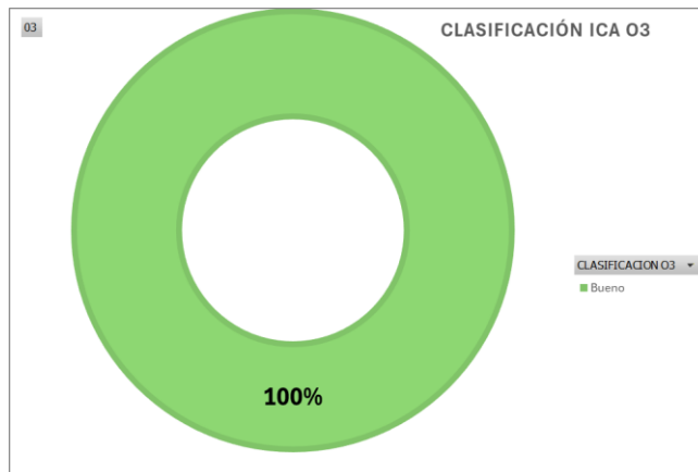
Gráfico 9. Índice de Calidad del Aire O 3 MAMONAL
